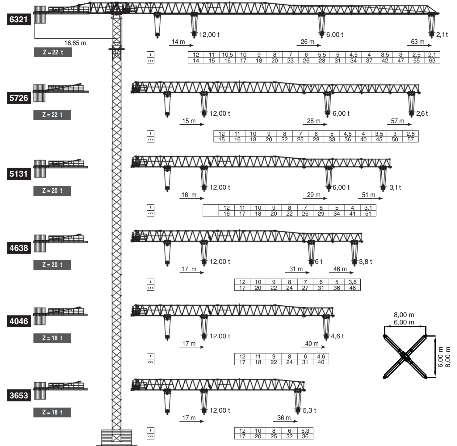
МАКСИМАЛЬНАЯ ВОЗМОЖНАЯ ВЫСОТА КРАНА С ПРИСТЕЖКОЙ – 200 МТ. 200 POSSIBLE MAX HEIGHT WITH ANCHORAGE FRAME
